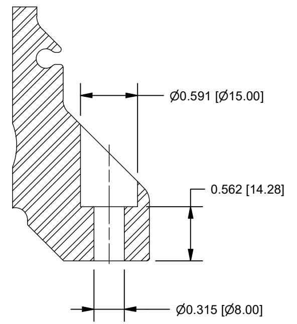
SECTION A-A TYP. 4 PLCS.
